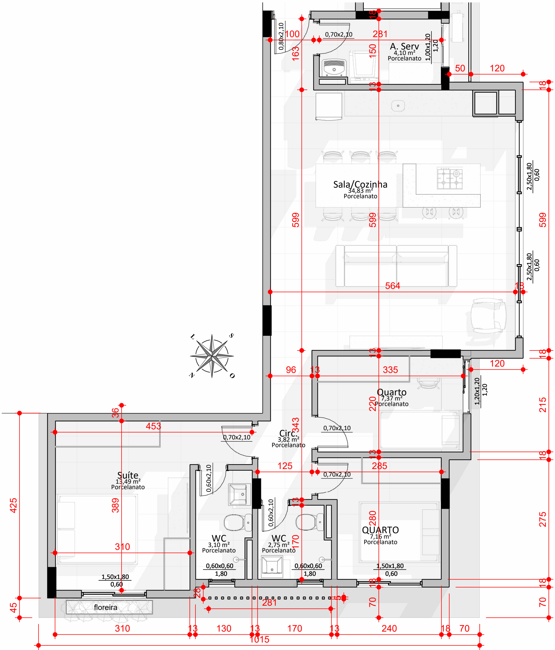
TIPO 1 89,54m²
