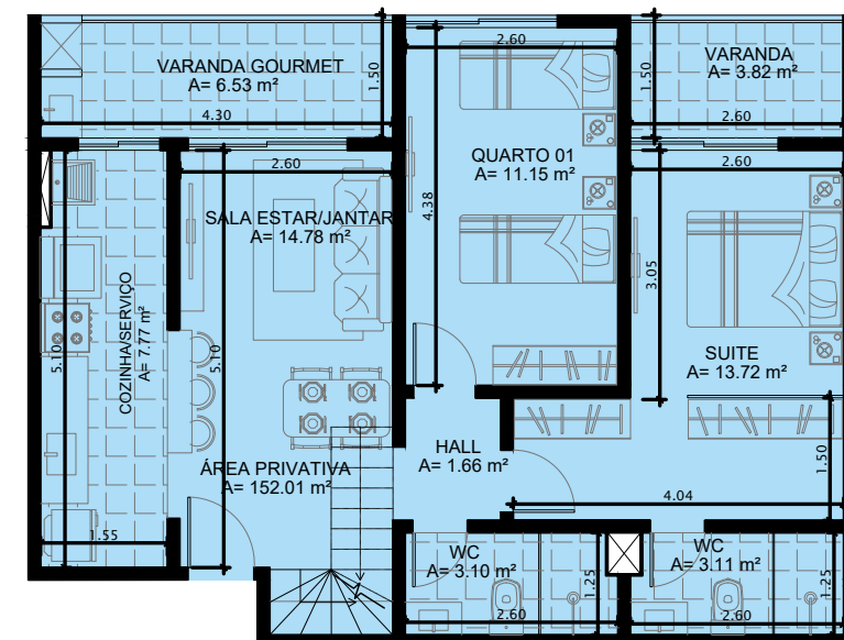
COBERTURA COLUNAS 1 E 2 - BLOCO 2
