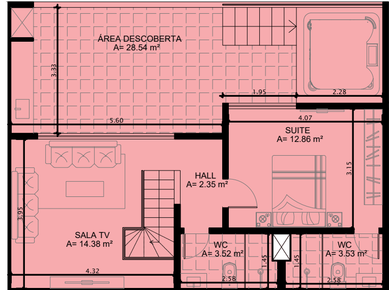
COBERTURAS COLUNA 3, 4, 5 e 6 - BLOCO 1 e 3 COBERTURAS COLUNA 3 e 4 - BLOCO 2
