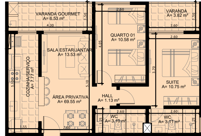
COLUNAS 1 E 2 - BLOCO 2 1º ANDAR
