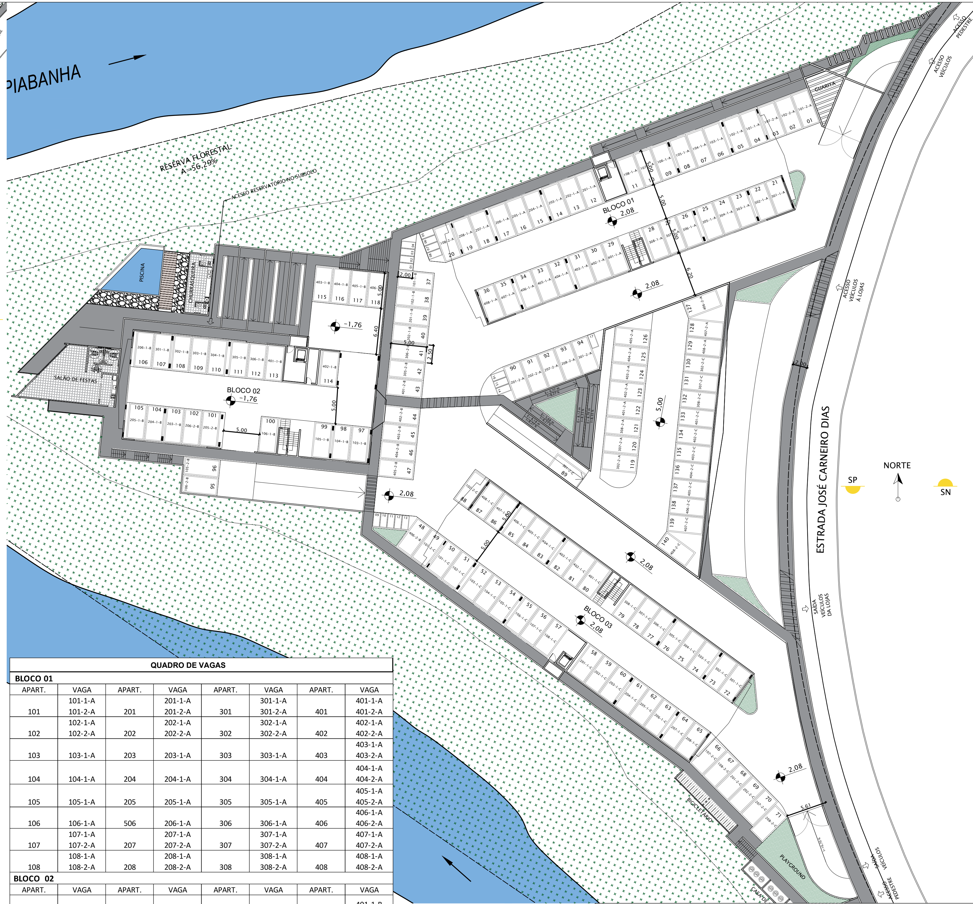
IMPLANTAÇÃO GARAGEM ESC: 1/300
