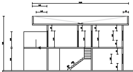
○ CORTE AA ESC.: 1/75
