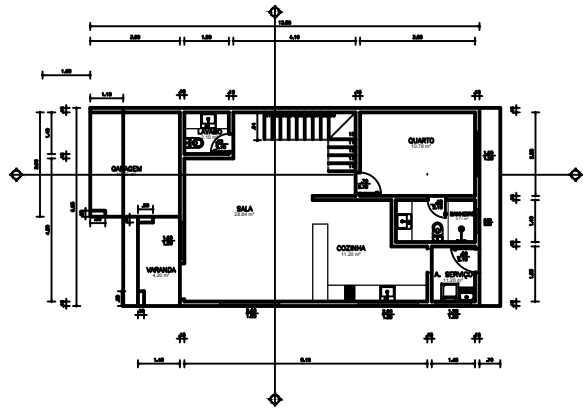
○ PAVIMENTO TERREO ESC.: 1/75
