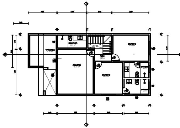
○ 2º PAVIMENTO ESC.: 1/75
