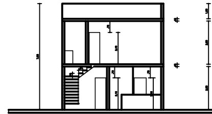
○ CORTE DD ESC.: 1/75
