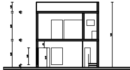
○ CORTE CC ESC.: 1/75
