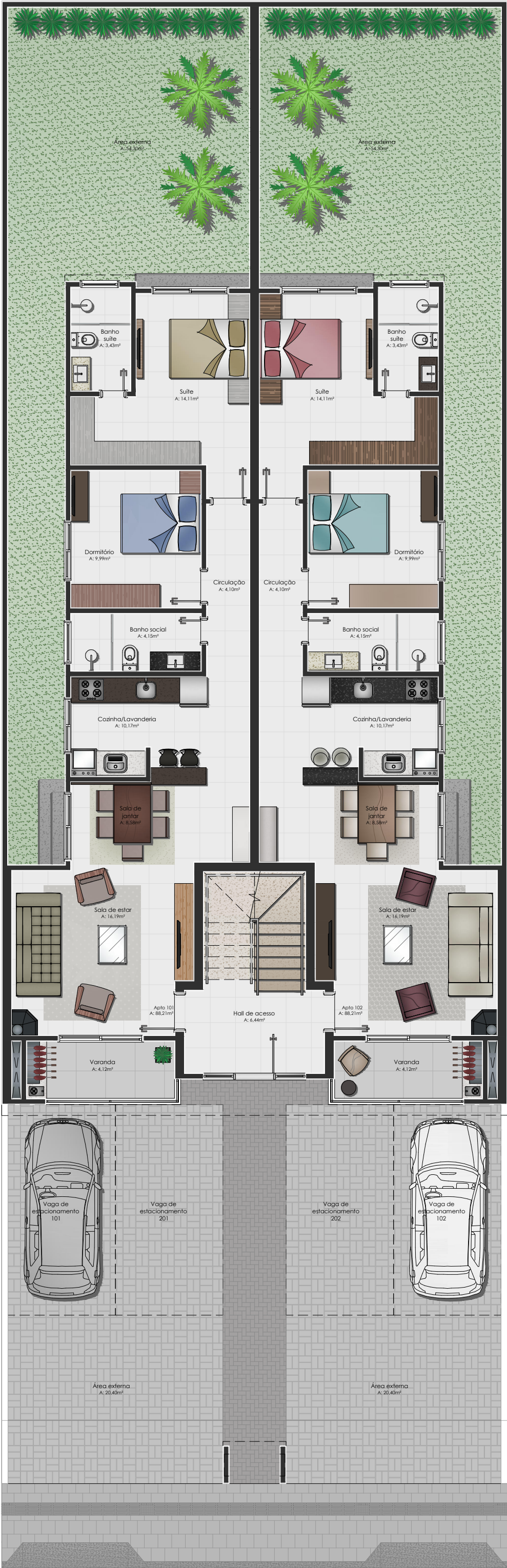
PLANTA TÉRREO
