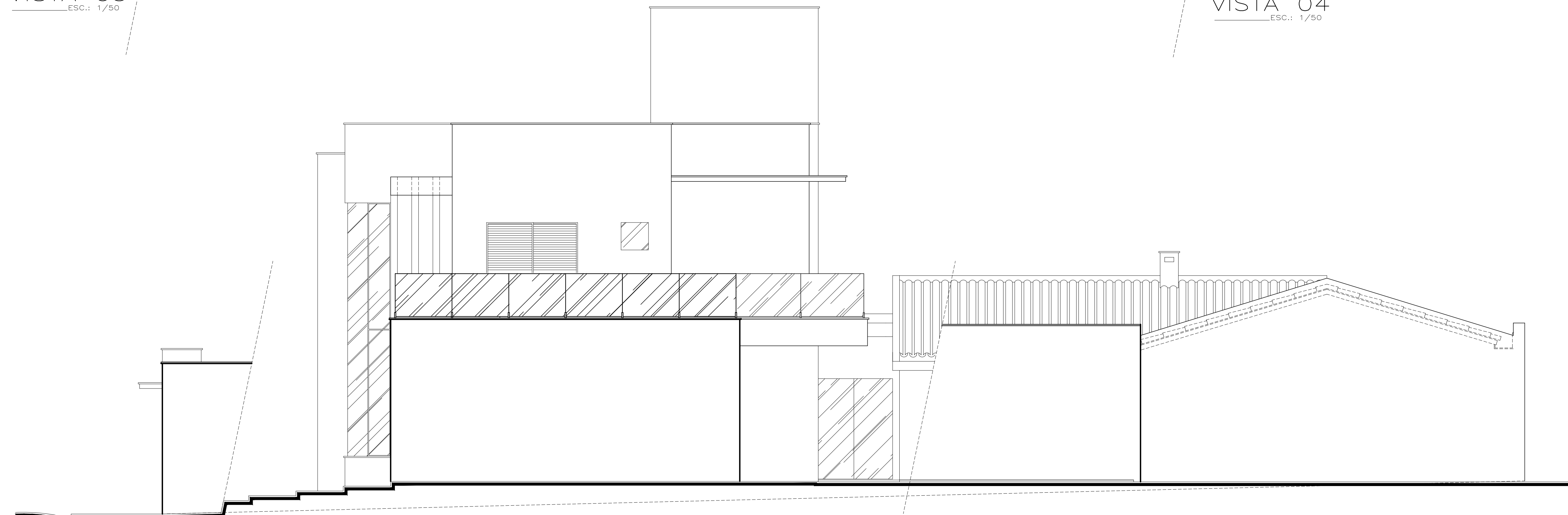
VISTA 05 ESC.: 1/50
