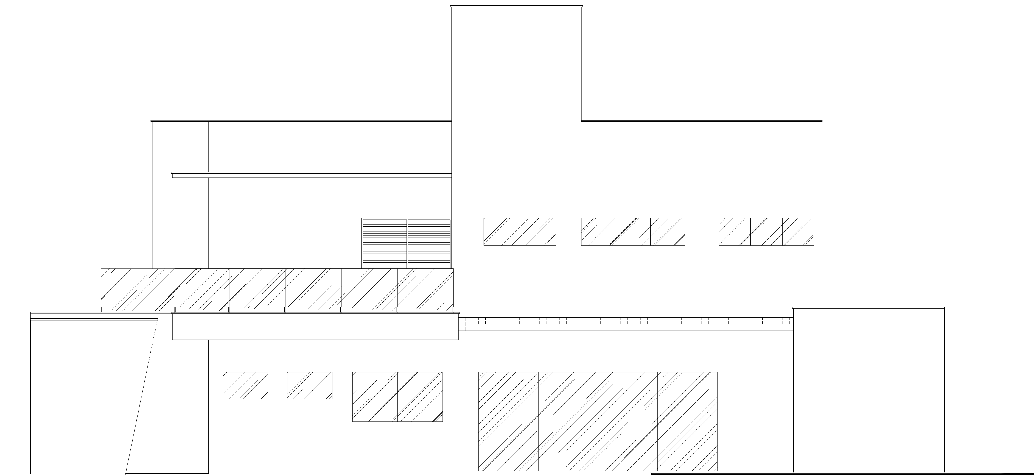
VISTA 04 ESC.: 1/50
