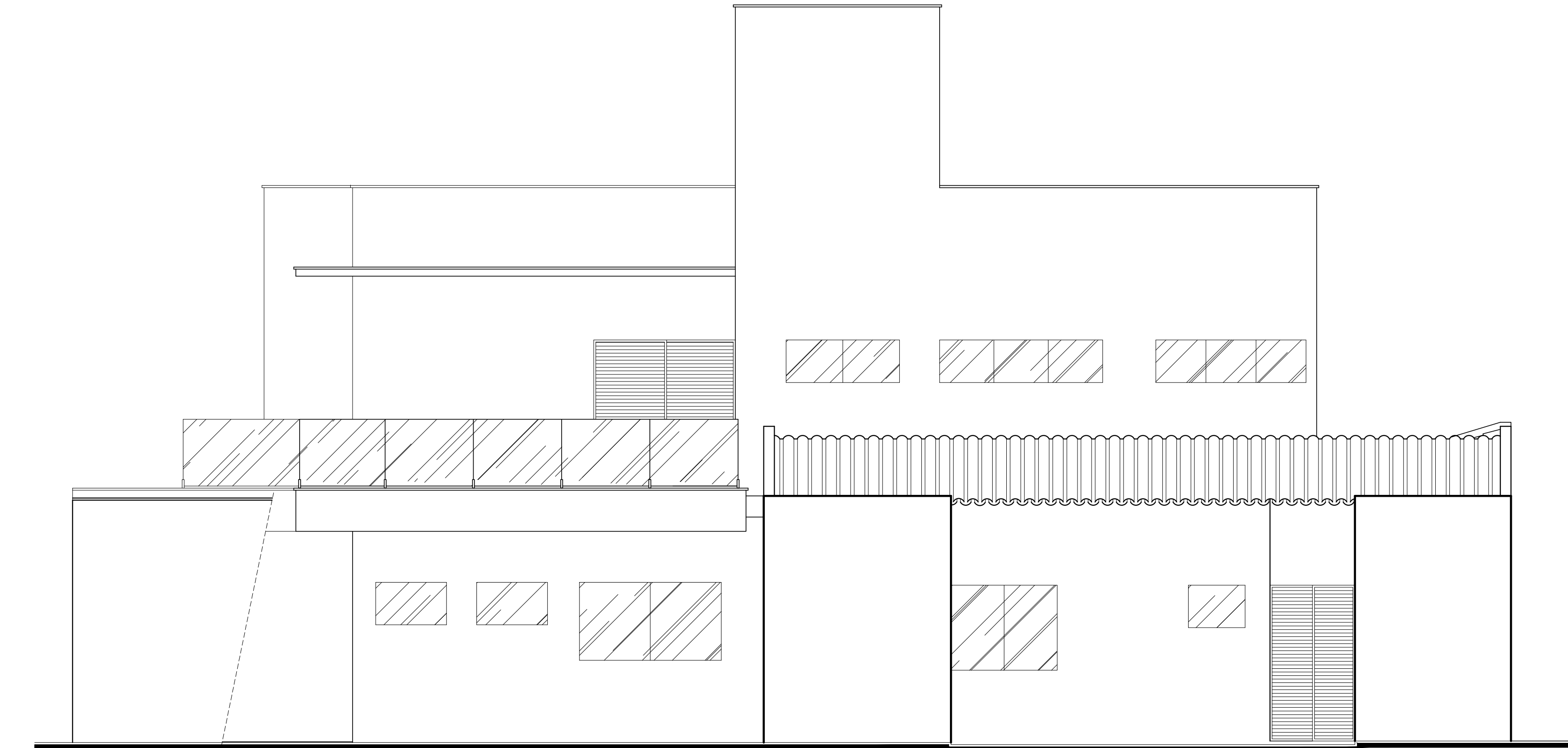
VISTA 03 ESC.: 1/50
