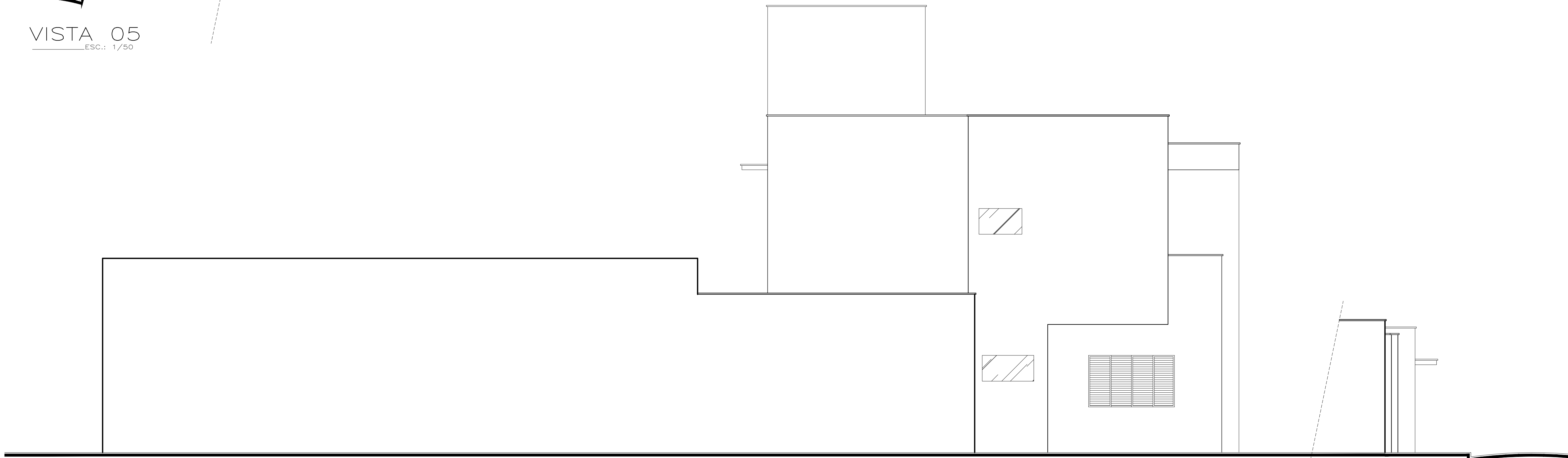
VISTA 02 ESC.: 1/50
