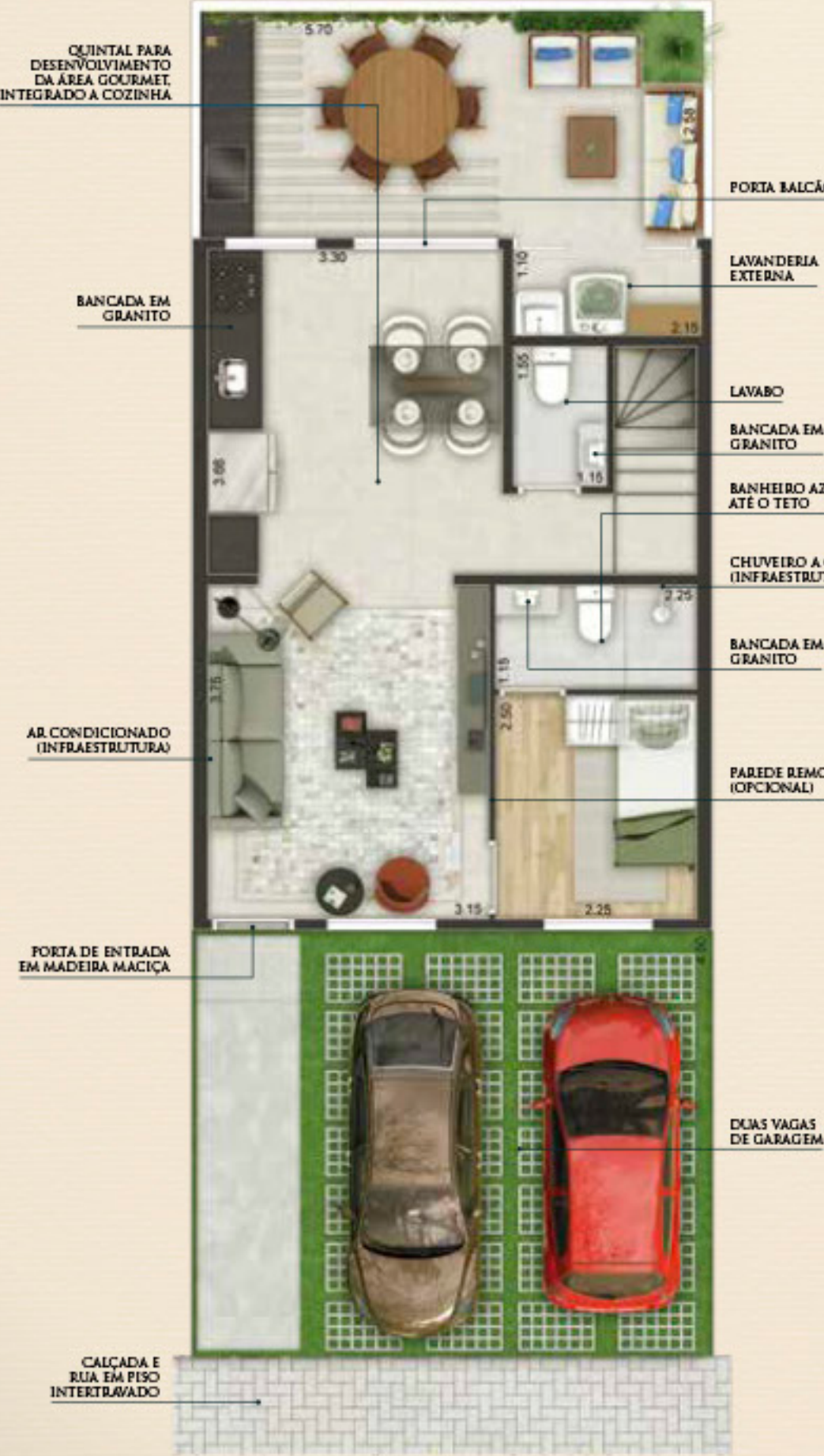
PISO TÉRREO
