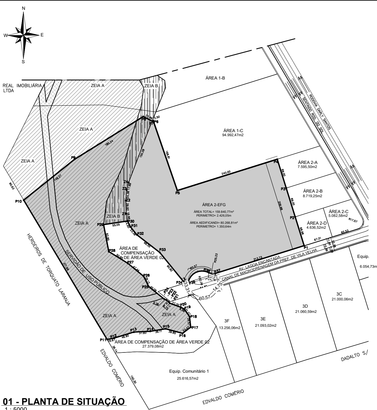
01 - PLANTA DE SITUAÇÃO 1 : 5000
